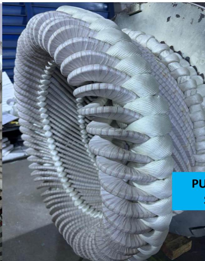
REBOBINADO MOTOR, MANTENIMIENTO MOTOR 5000HP PETROPIAR
